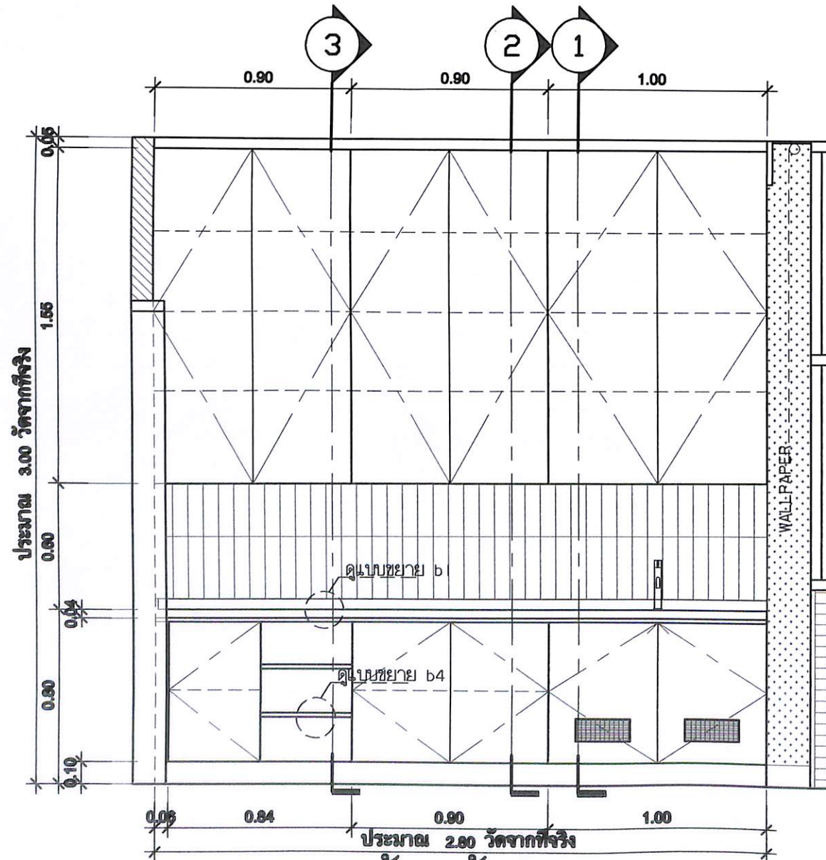
รูปด้านหน้า BF4.3
