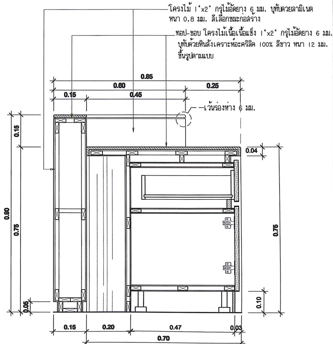
รูปตัด BF2
