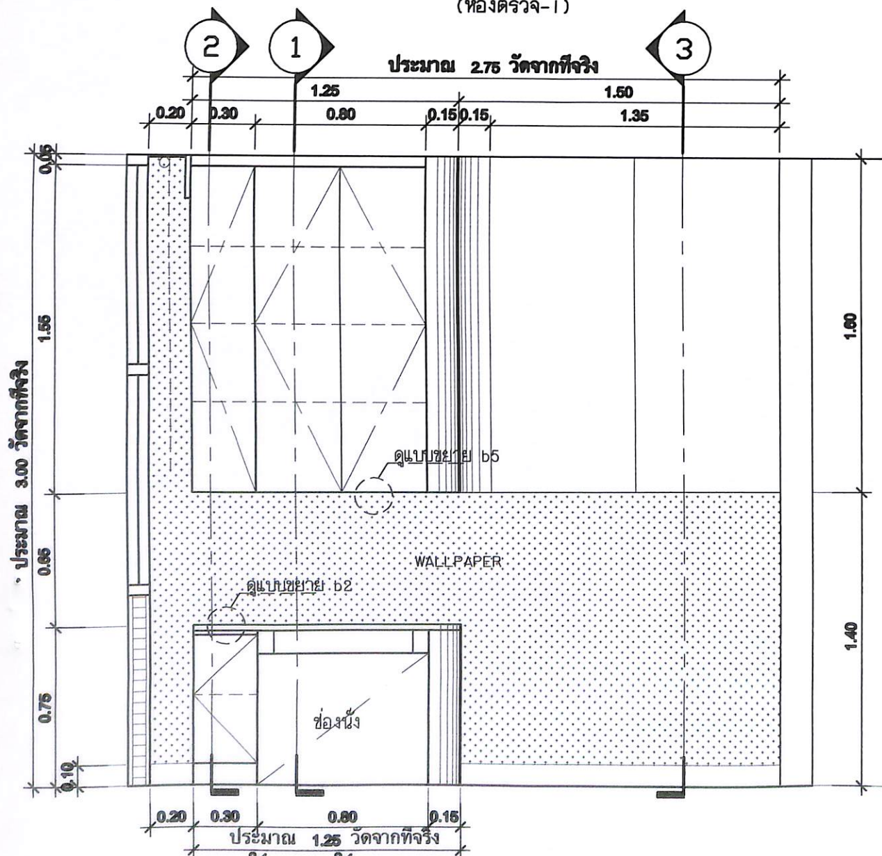
รูปด้านหน้า BF6.1
