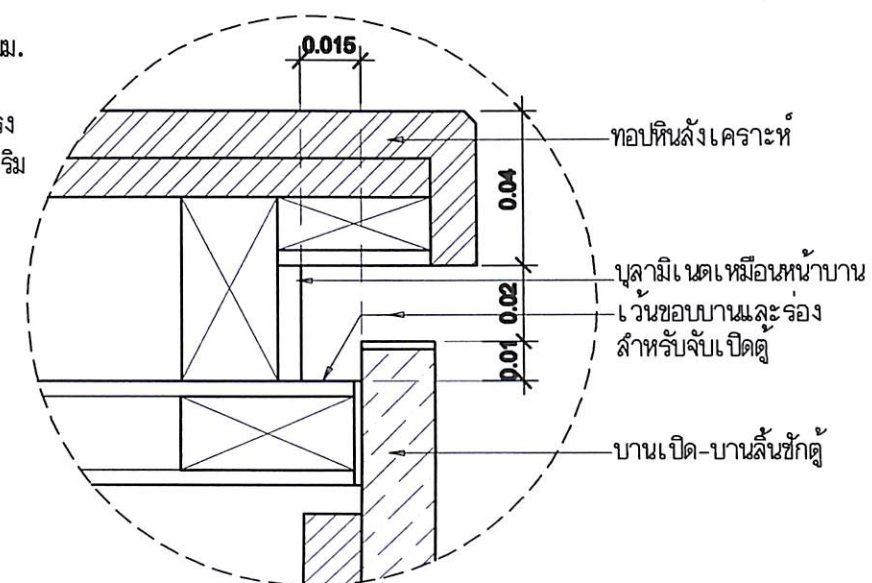
แบบขยาย b1 มาตราส่วน 1:2
