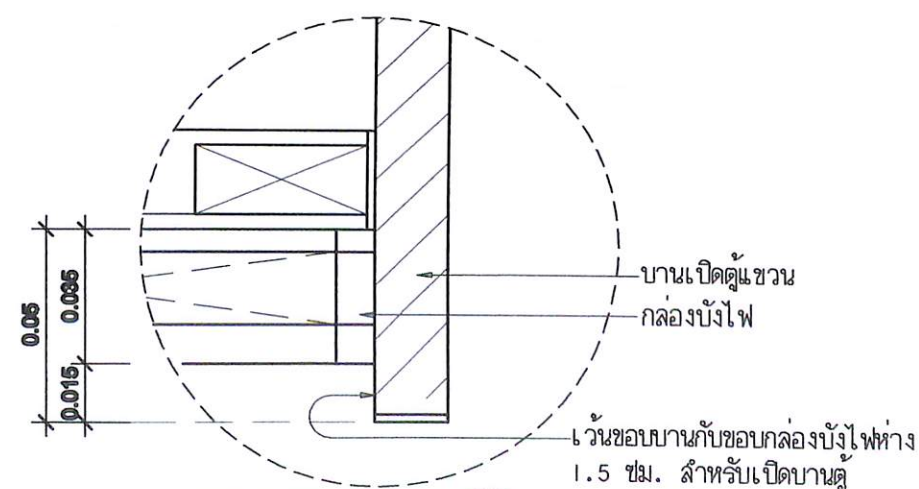
แบบขยาย b5 มาตราส่วน 1:2
