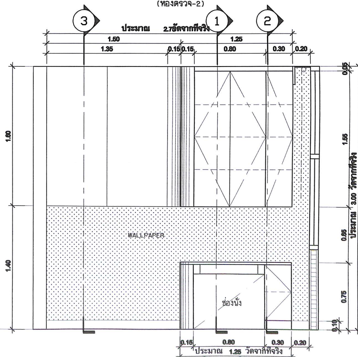
รูปด้านหน้า BF6.2
