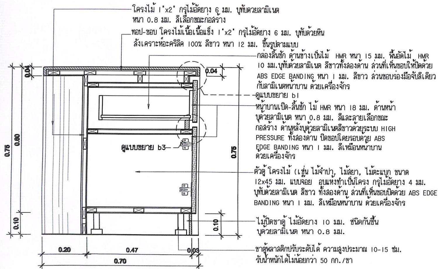
รูปตัด BF2
